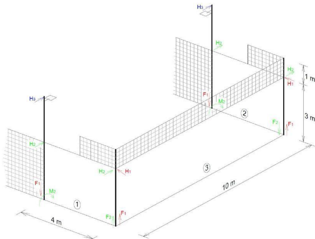
Figuur 11: reactiekrachten aangegeven in 3d model panoramakooi
