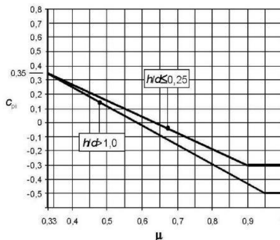
Figuur 7.13 — Inwendige drukcoëfficiënten voor gelijkmatig verdeelde openingen
