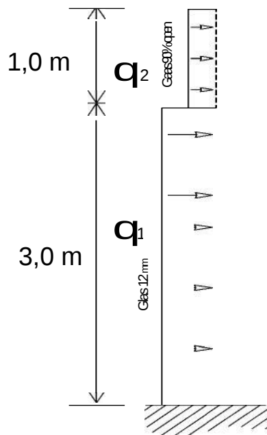
Figuur 12: belastingschema framekooi of pilaar systeem kooi
